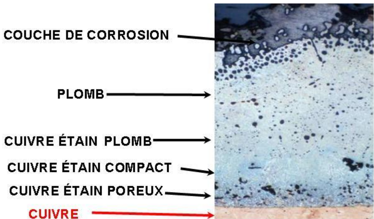
Figure 5a : Microstructure de la médaille au niveau de l'endommagement
