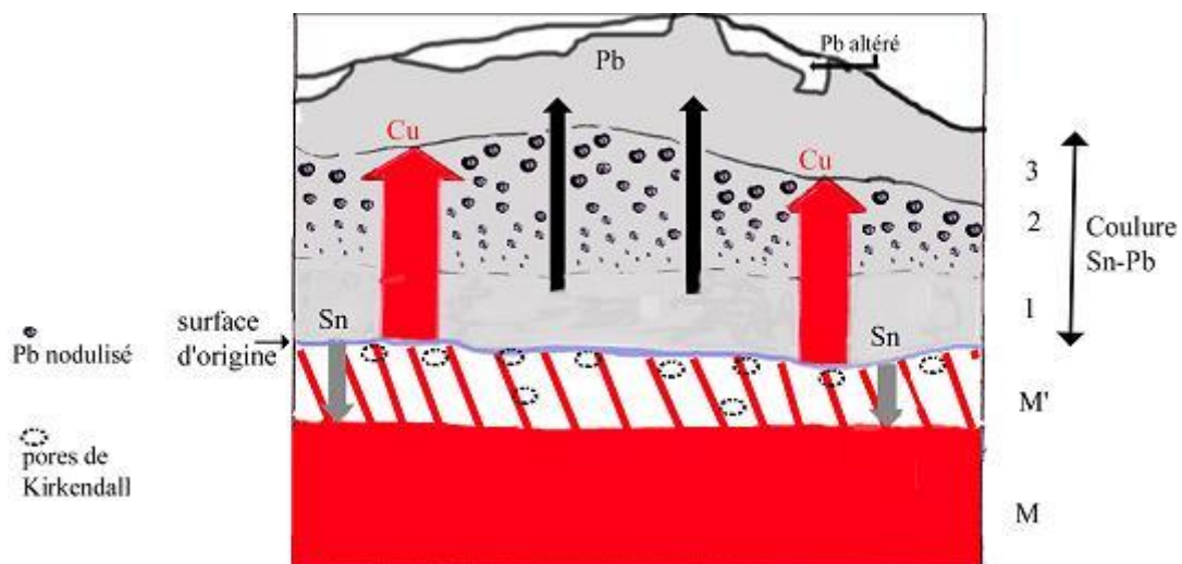
Figure 5b: Schéma du mécanisme diffusionnel
